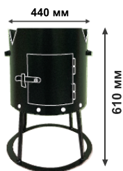
ПЕЧЬ под КАЗАН 16 литров
