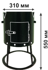
ПЕЧЬ под КАЗАН 6 литров
