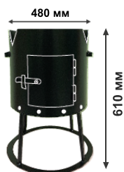
ПЕЧЬ под КАЗАН 22 литра
